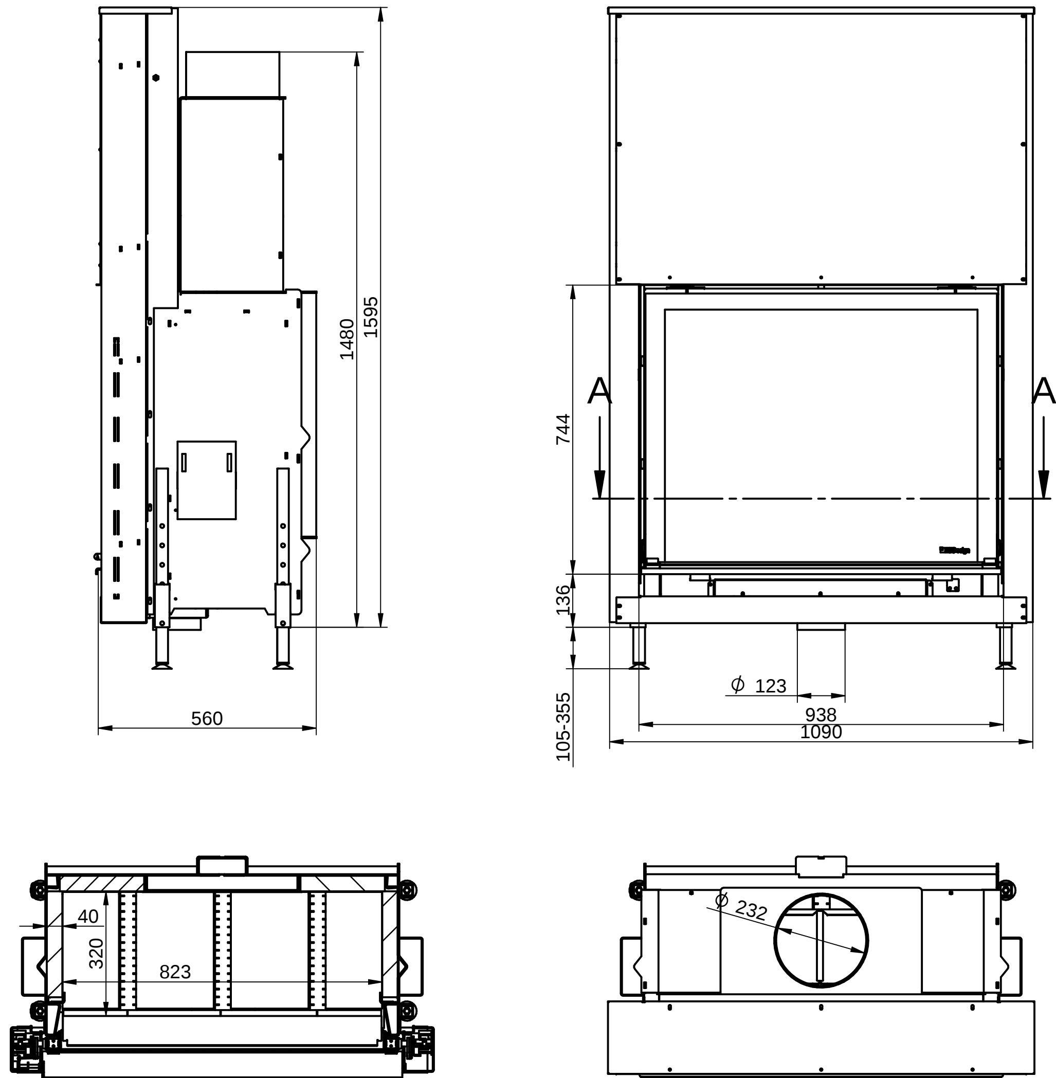
SECTION A-A
